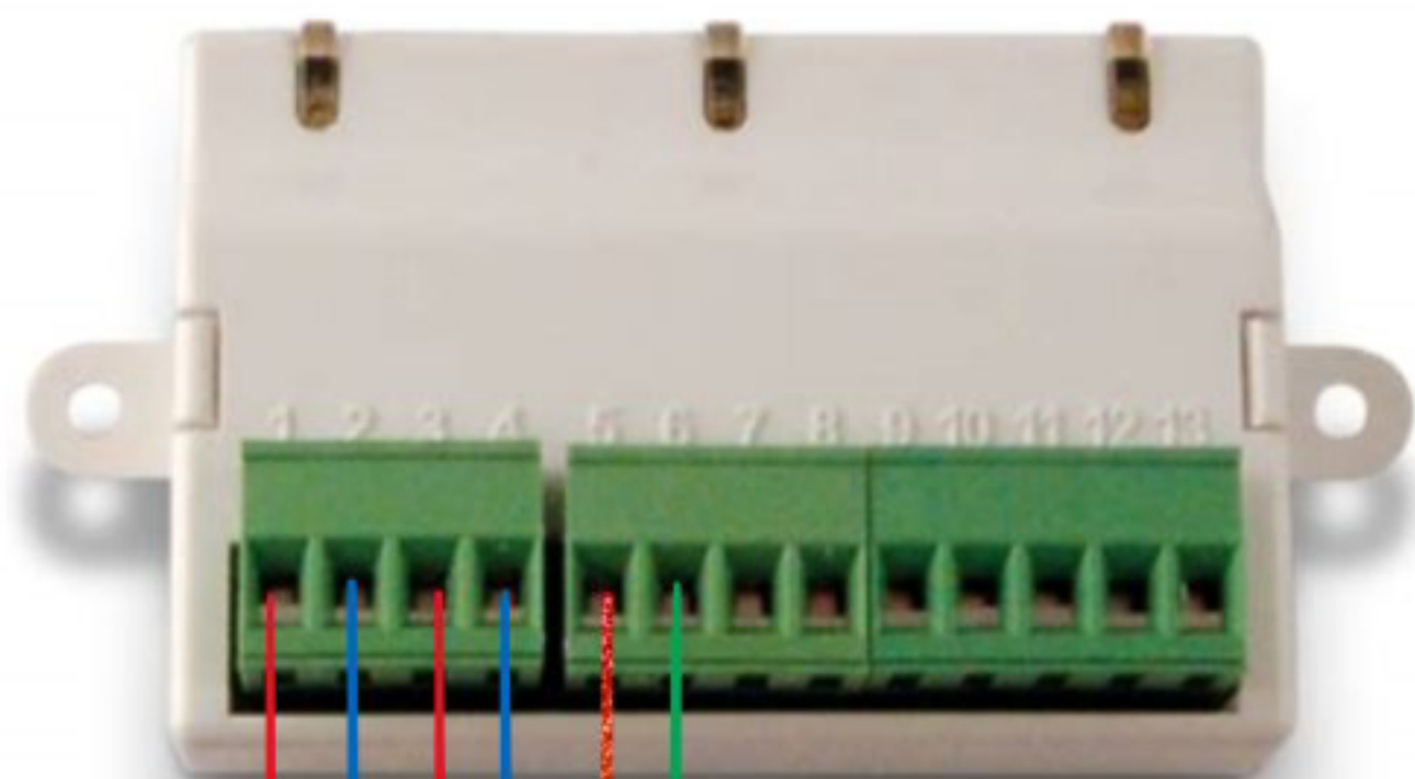
INIM EM411R alaosoiteyksikkö
