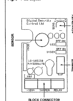
Fig. 5 - PCB Layout
