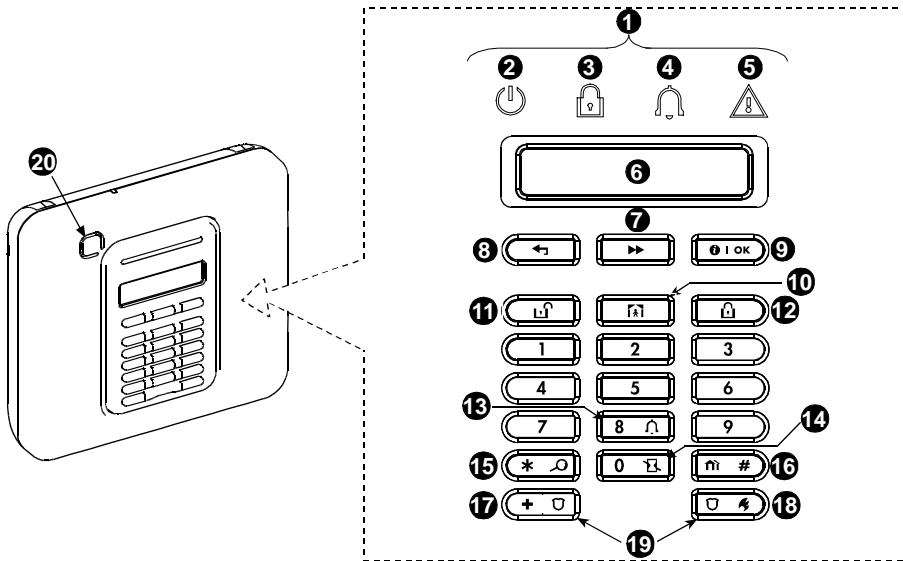
Kuva 1a. WP8010-järjestelmän ohjaimet ja merkit
