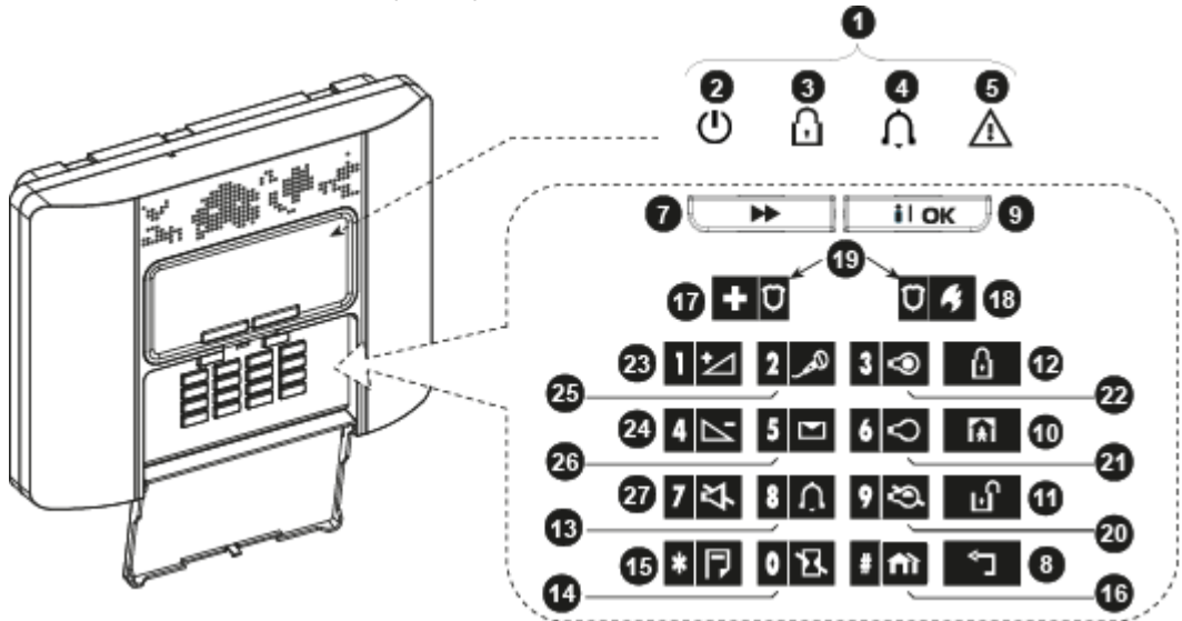
Kuva 1b. WP8030-järjestelmän ohjaimet ja merkit
